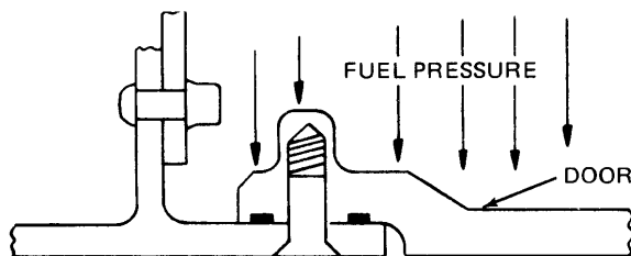
Figure 6-6. Plug Door
