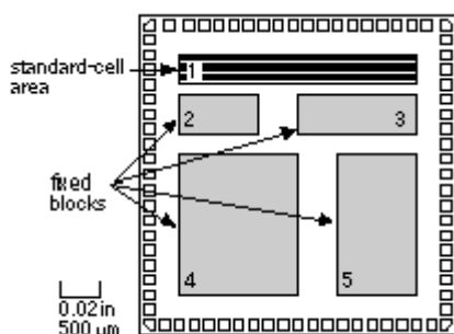
Figure C-7: ASIC Die
