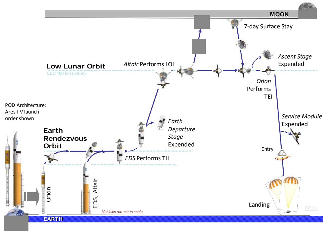
FIGURE 3.1.1-1 LUNAR SORTIE CREW DRM
