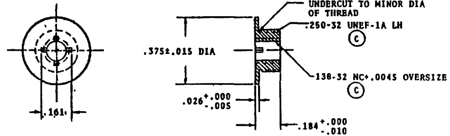
-3, -6 FLANGE
