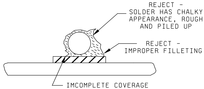
FIGURE 2017-23e. Solder criteria.
