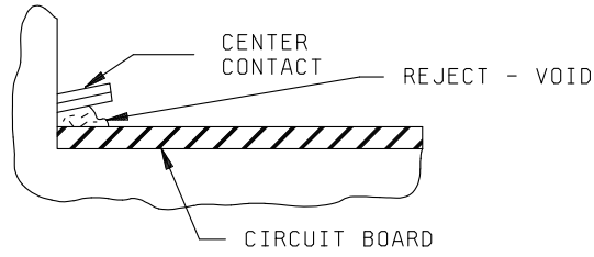
FIGURE 2017-23a. Void criteria.
