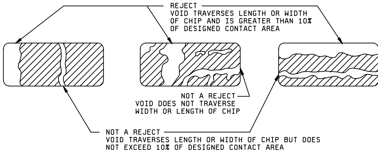
(b) VOIDS
