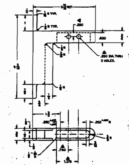
1 DETAIL 14E TANG MATL. 304 L NO. REQD: 1 PER STYLE
