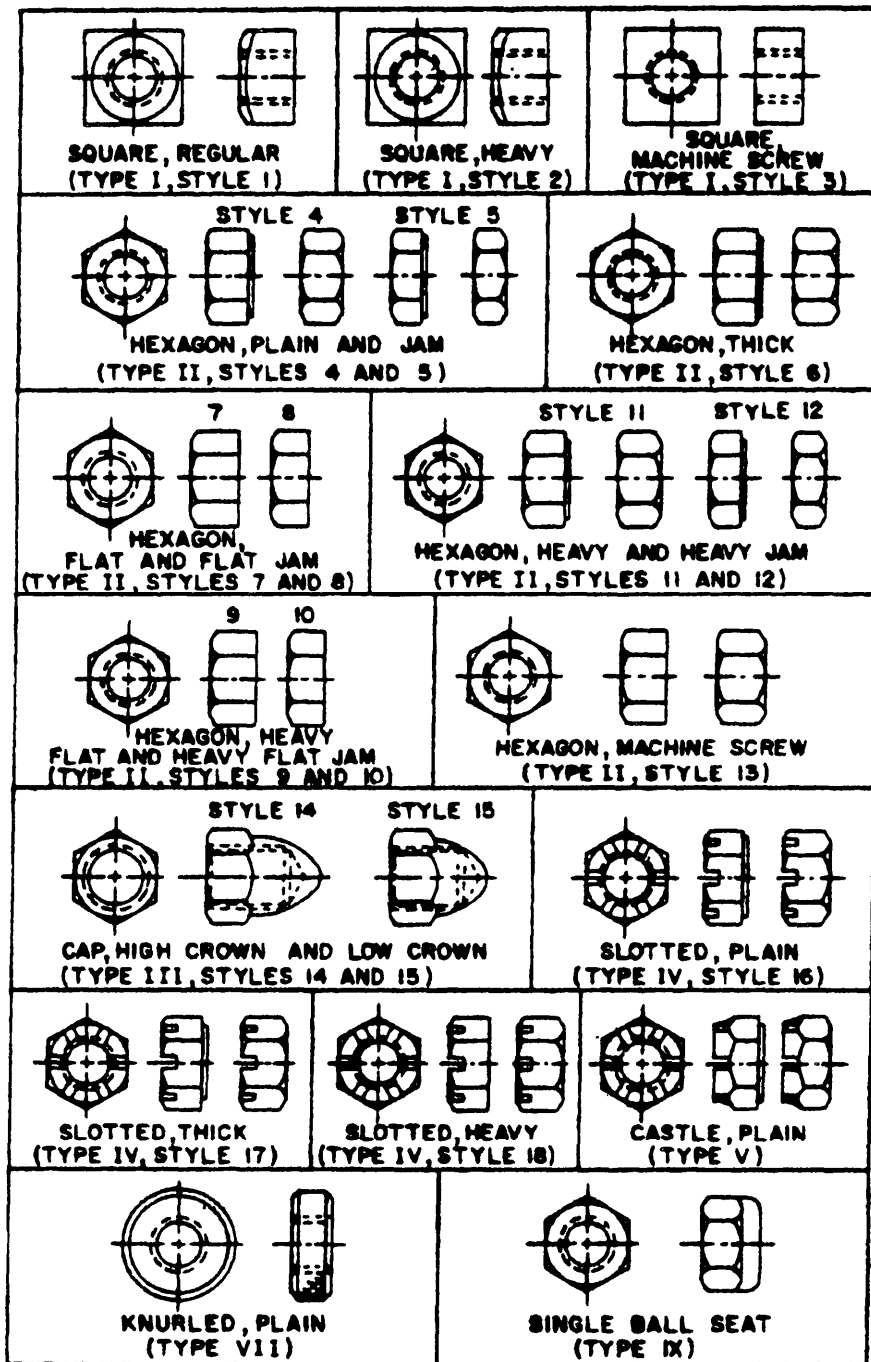
FIGURE 1 (CONTD) - NUTS
