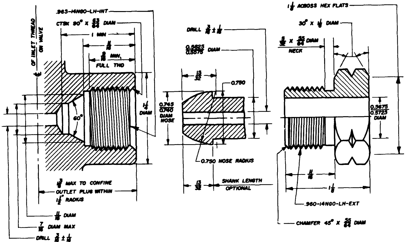
HEX NUT NO. 594
