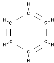
BENZENE RING
