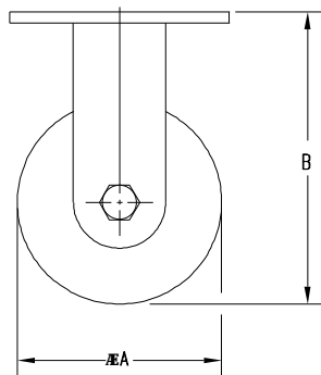
FIG. 1. RIGID CASTER
