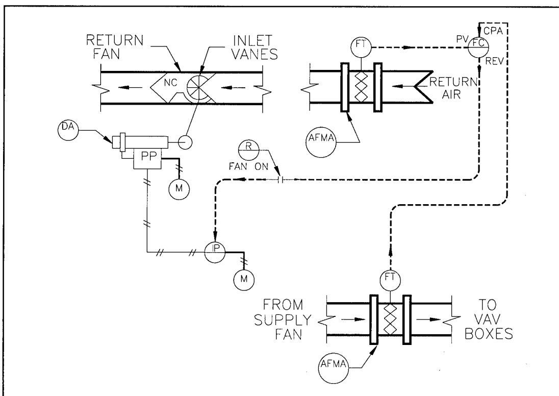
Figure 24. Return fan volume control loop.
