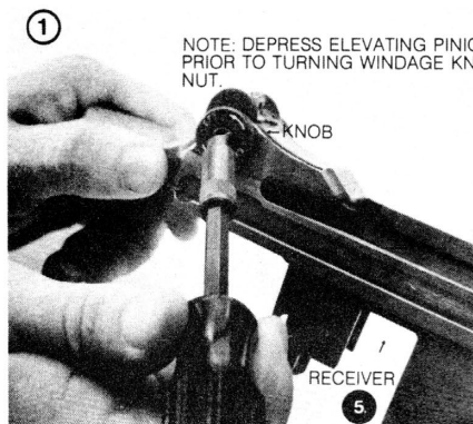
LOOSEN/TIGHTEN NUT.
