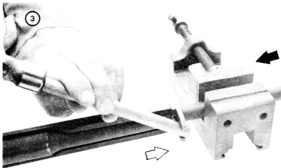
LOOSEN/TIGHTEN BAND
